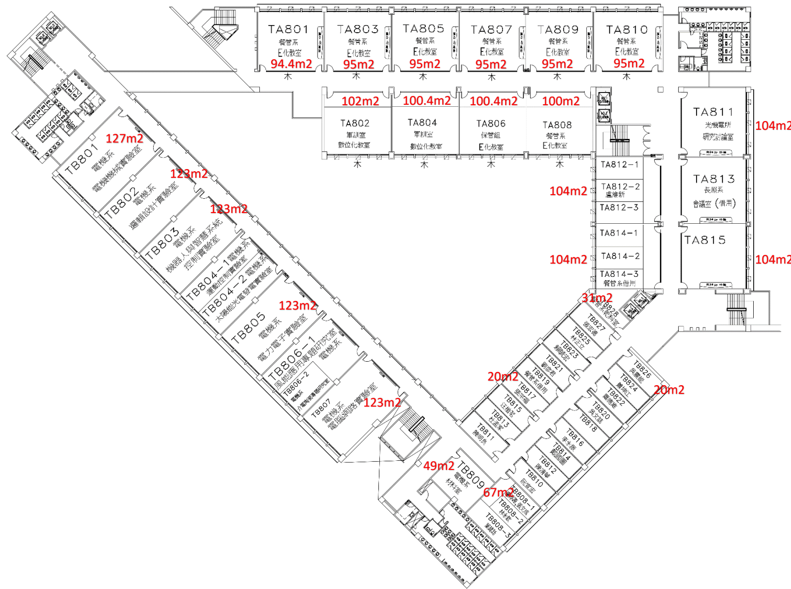
花明樓捌層平面圖
