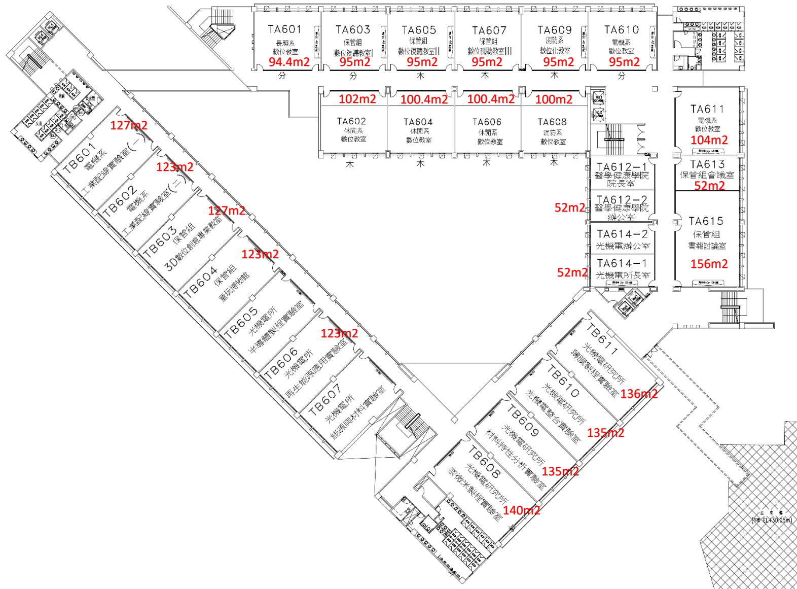
花明樓陸層平面圖
