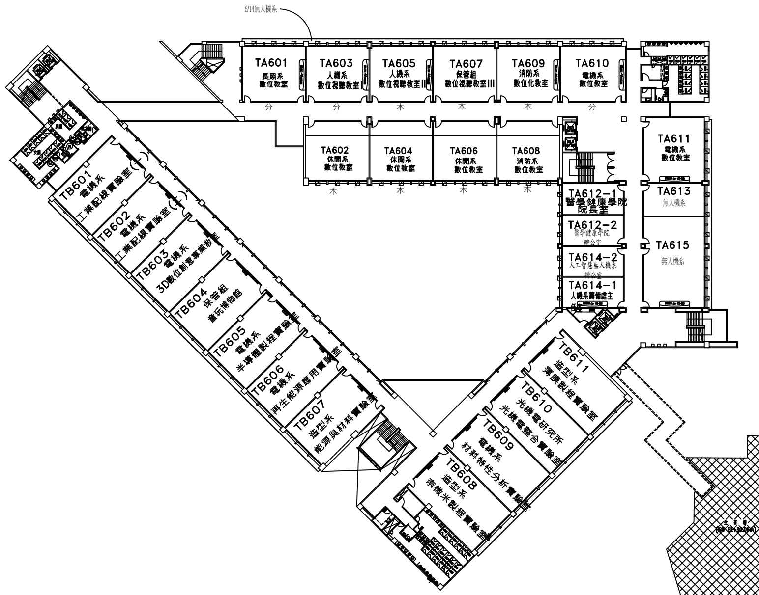
花明樓陸層平面
