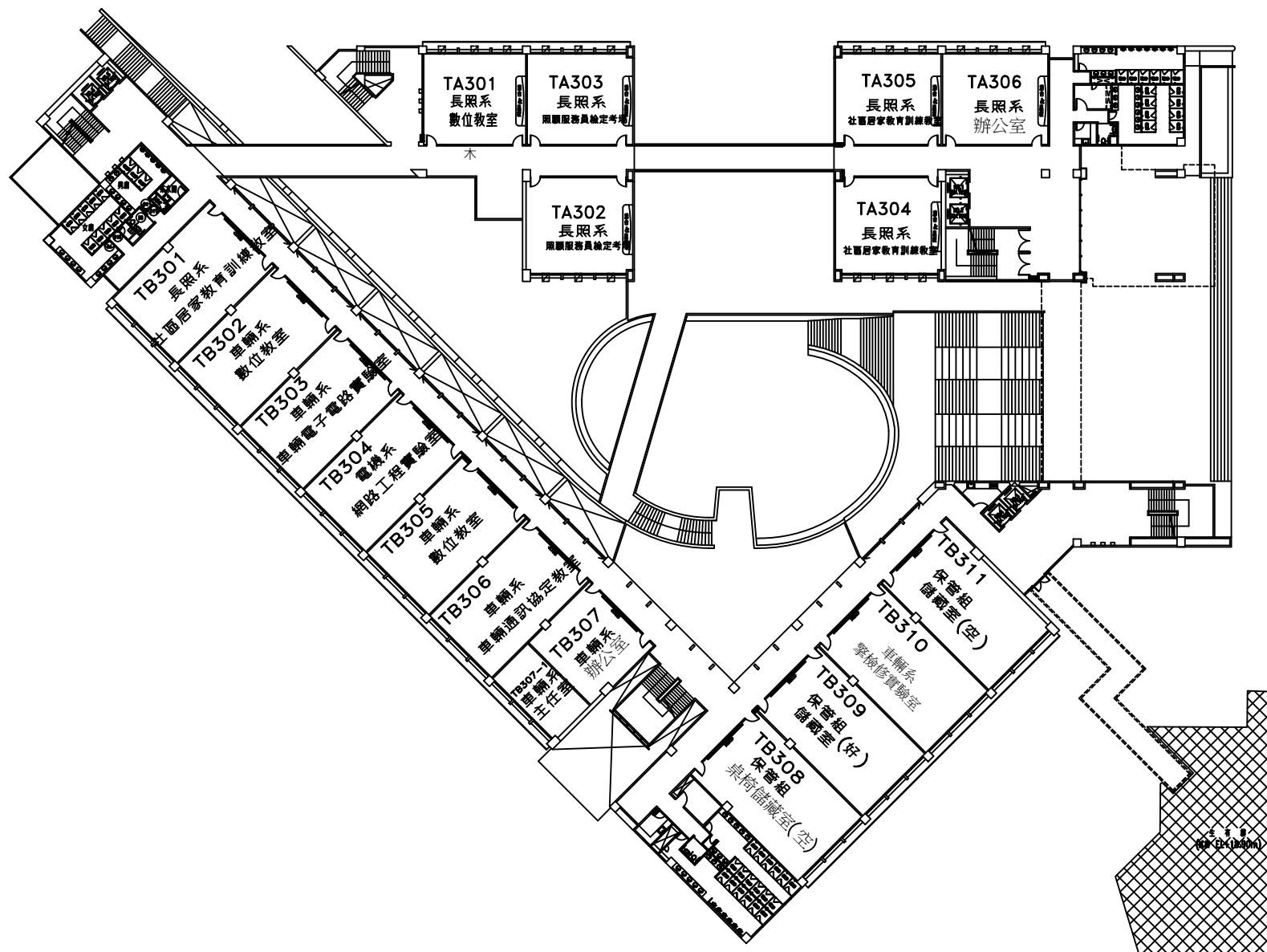
花明樓參層平面
